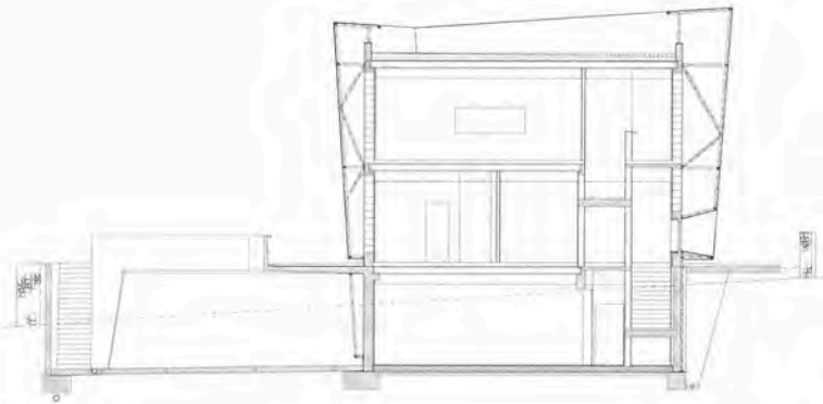
Schnitt Section
