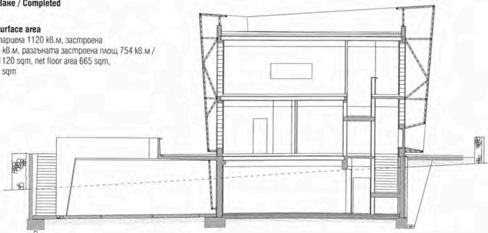
Разрез / Section
